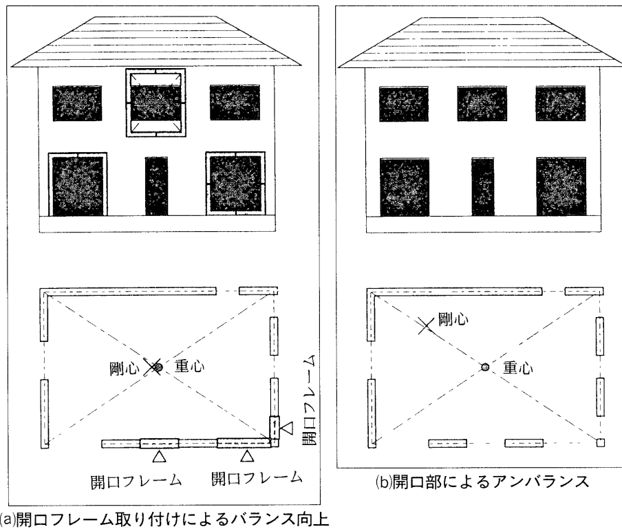
図6 木造建築物の耐震性バランスの状況
