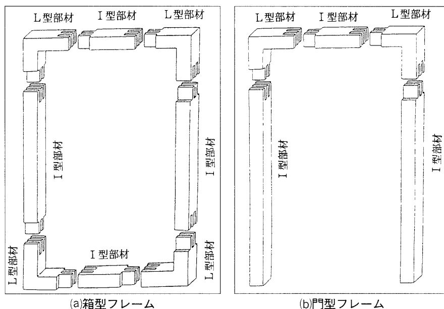
図1 木造開口フレームの構成
