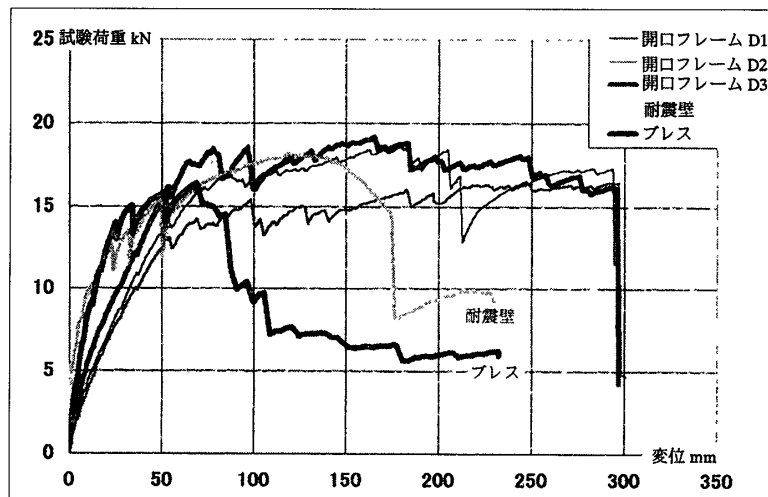
図8 木造開口フレームの試験結果
