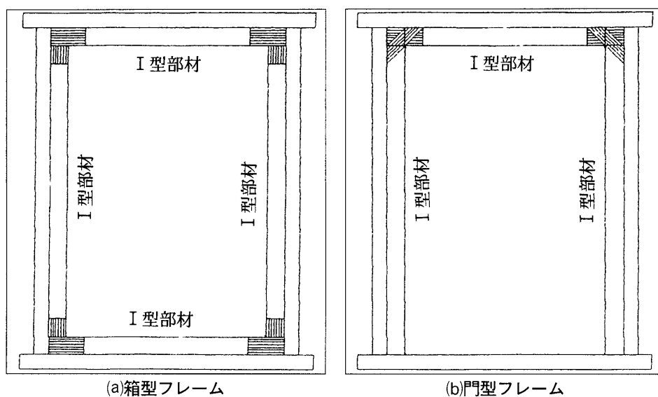
図2 木造開口フレームの構成
