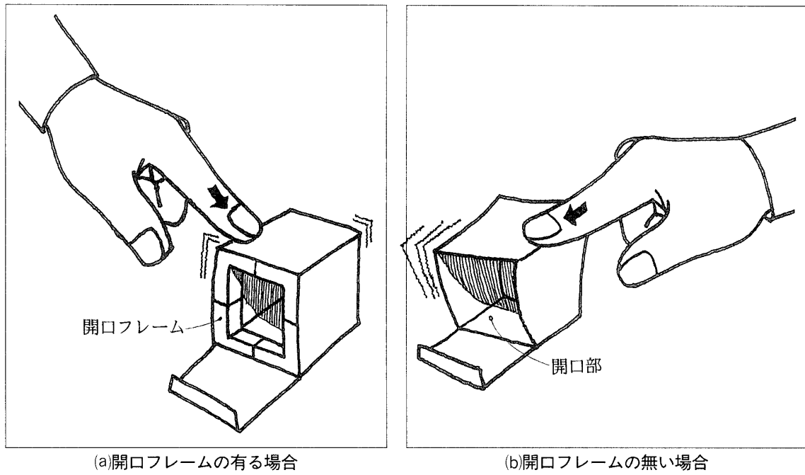
図5 建築物変形の模擬図
