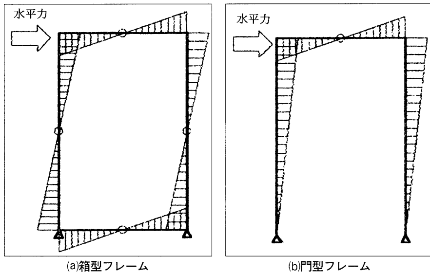
図3 木造開口フレームの曲げモーメント
