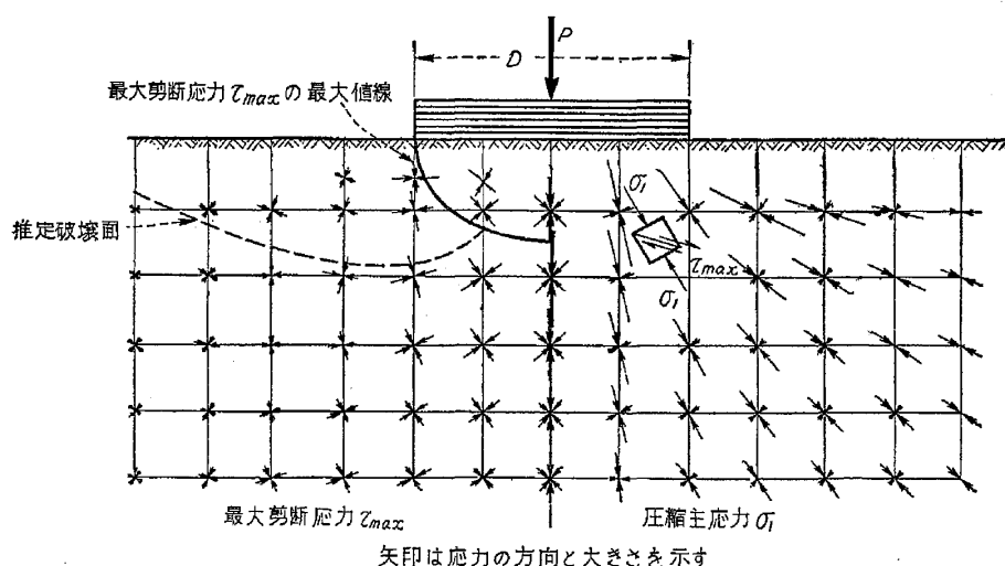
図 1 円形載荷面の下の応力分布
