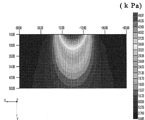
図 22 FEM 解析結果 (動的)
