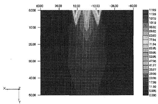
図 24 FEM 解析結果 (静的)
