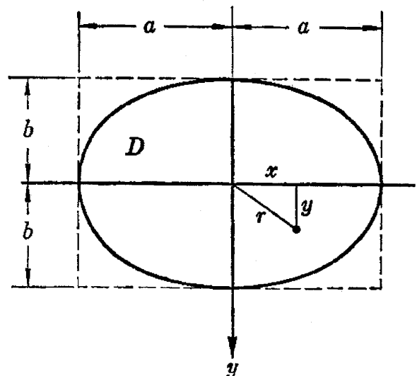
図8 楕円形の載荷板の座標系
