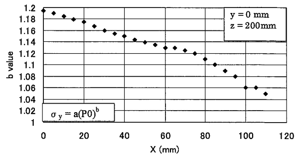
図 3 測定位置による載荷圧依存性
