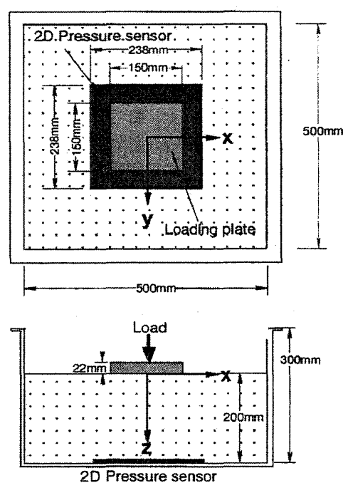
図 2 二次元圧力シート
