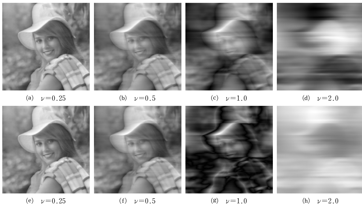
図 10 I_{\nu}^{\alpha} f_E(x, y) の (a)–(d) 線形濃度表示, および (e)–(h) 絶対濃度表示
