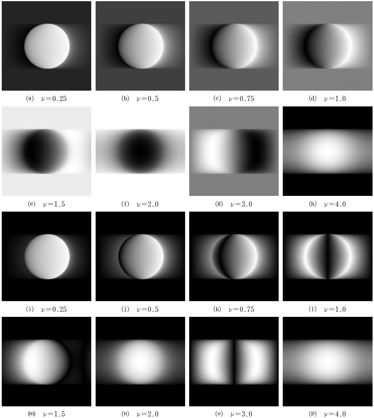
図5 I_\nu f_D(x, y) の (a)–(h) 線形濃度表示, および (i)–(p) 絶対濃度表示
