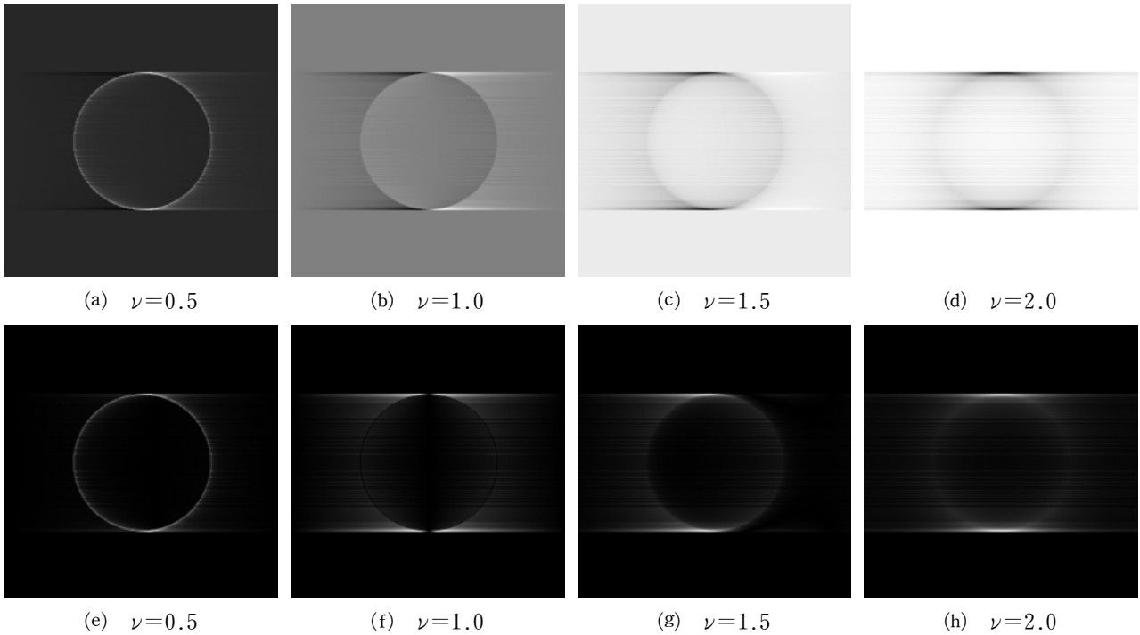
図 8 I_x^\nu f_c(x, y) の (a)–(d) 線形濃度表示, および (e)–(h) 絶対濃度表示
