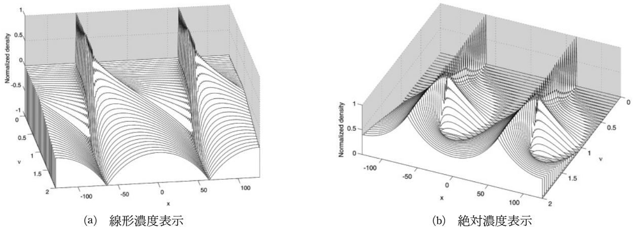
図 9 I_x^\nu f_c(x, y) の中心水平断面の \nu に対する変化
