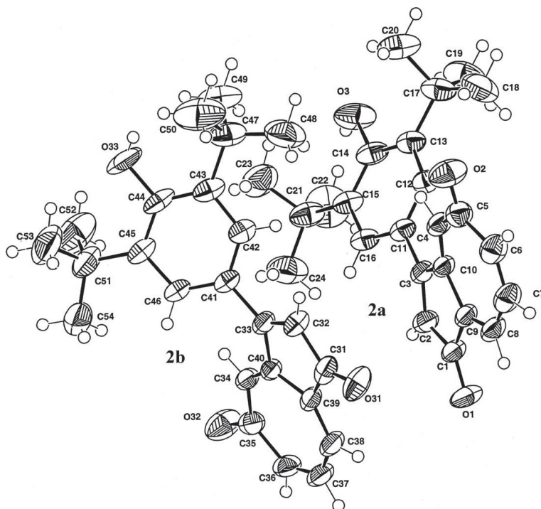
Fig. 3. ORTEP diagram of 2 .
