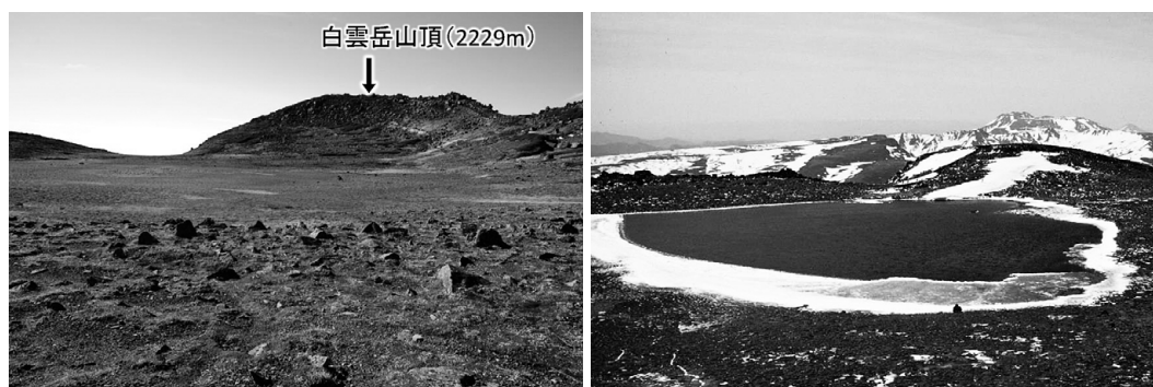
写真1 白雲岳火口原 右の写真は火口湖出現時に北側から火口原を見たもの
