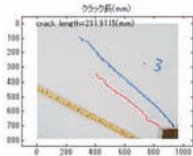
(c) ひび割れ長 (232mm)
