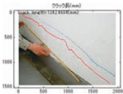
(c) ひび割れ長 (1342mm)
