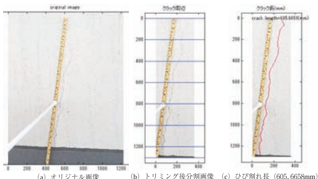
図-12 統計処理実施ひび割れサンプル (有効画素数2304×1704pixel)
