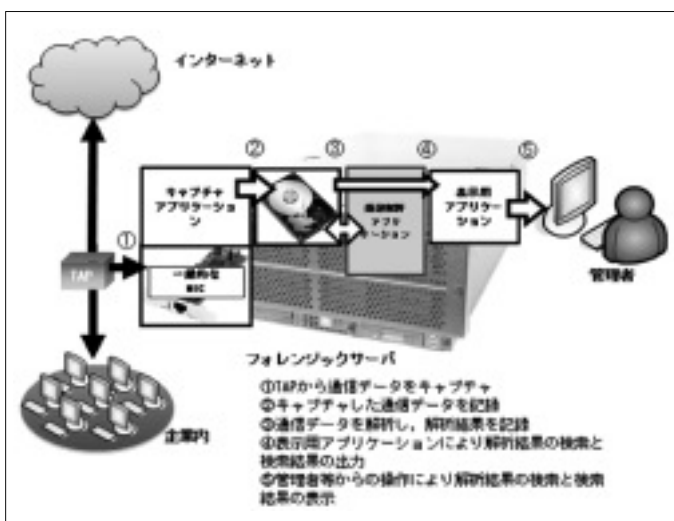
図6 プレイバック直前での解析処理
