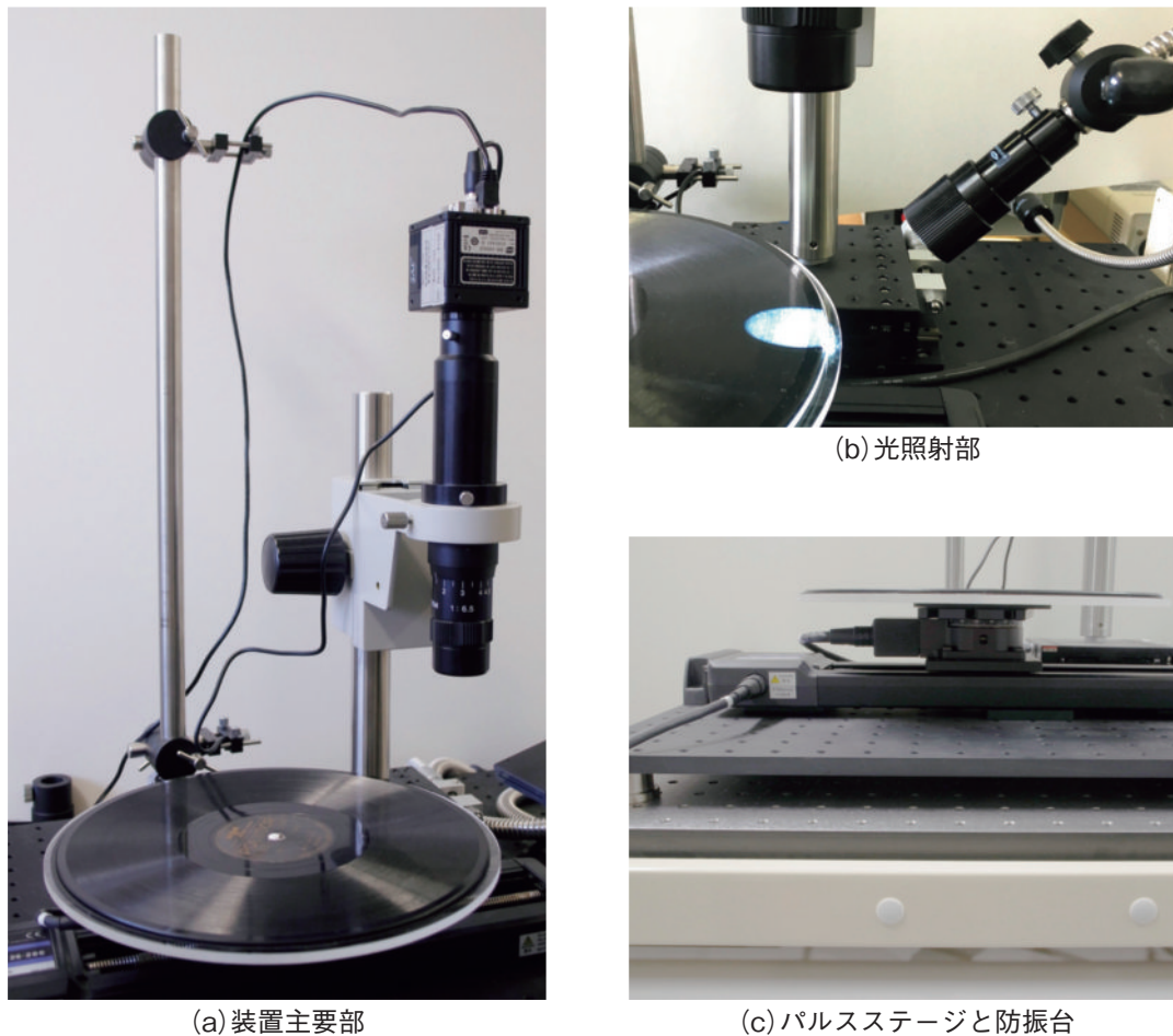
図1 実験装置
