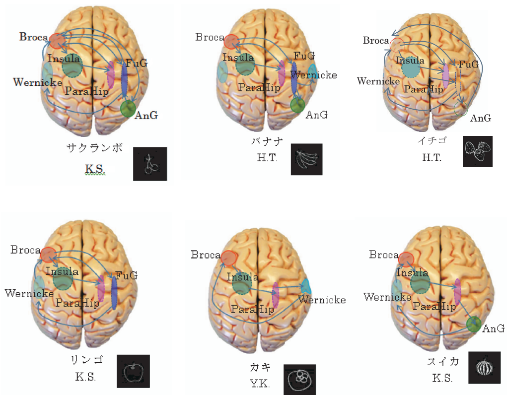
図3 後半処理の脳内活動経路比較
