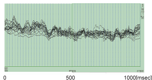
図2 被験者KSのERPデータ
