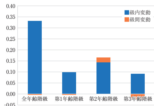
図7(a) 基準時点における要因分解図(ジニ係数)
