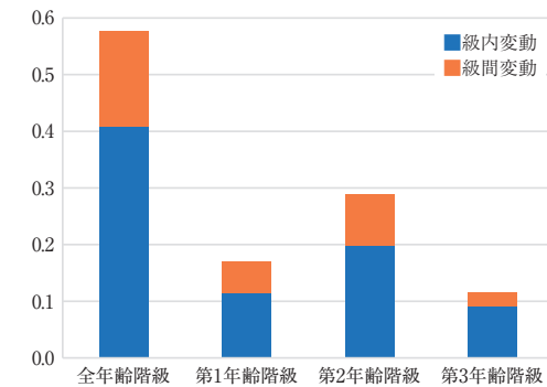
図 6 (a) 基準時点における要因分解図 (変動係数)
