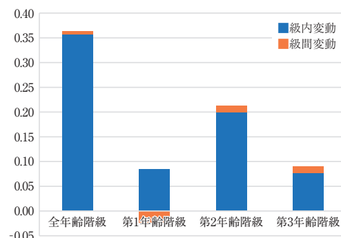
図7(b) 比較時点における要因分解図(ジニ係数)
