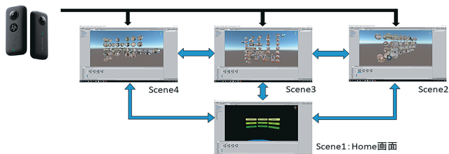
図7 画像データが多い場合のシーンの分割
