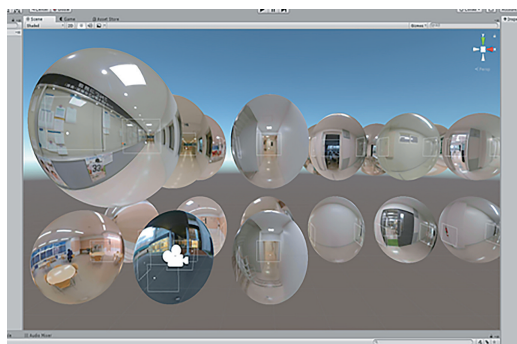
図6 Unityシステム内での複数360度カメラ画像の球体への写像
