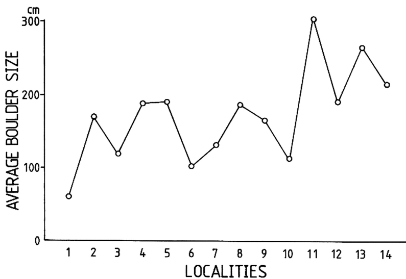
図10 各地点における平均岩塊長径 (高橋, 1985b より)
