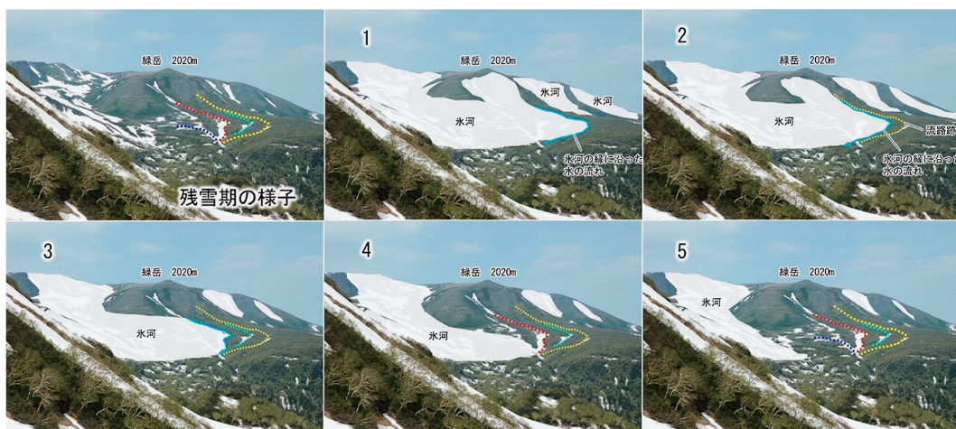
写真 18 緑岳南斜面における水河縮小とそれに伴う水河縁辺水路の形成（写真中の水河は仮想）
