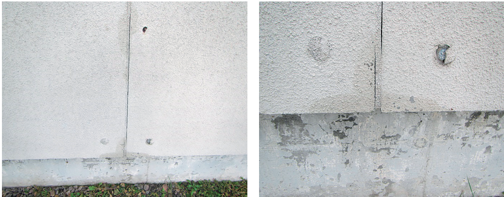
写真3 複合板間シーリングの切れからの水の浸入と滲出、ファスナー頭部における剥離 (右は接写)
