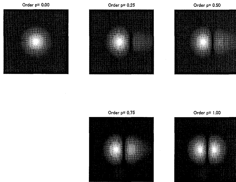
図3 0.25 \leq p \leq 1.0 におけるガウス分布画像の非整数次微分。画像サイズはおおの512×512。表示はその中央部分の128×128の領域。 p = 0.00 は原画像パターン。
